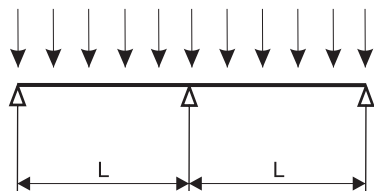
Двухпролетная схема нагружения
