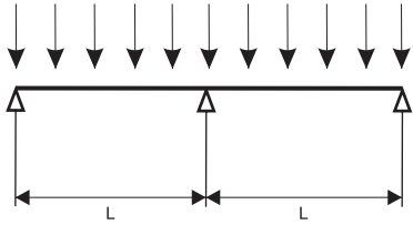
Двухпролетная схема нагружения
