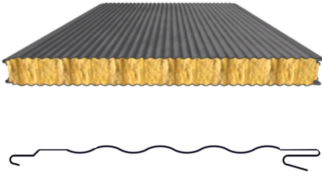
Волнообразная поверхность (микропрофилирование)
